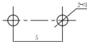
印制线路板开孔 P.C.B. HOLE DETAIL
