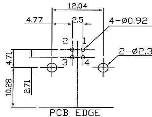
PCB EDGE (COMPONENT SIDE) PCB LAYOUT
